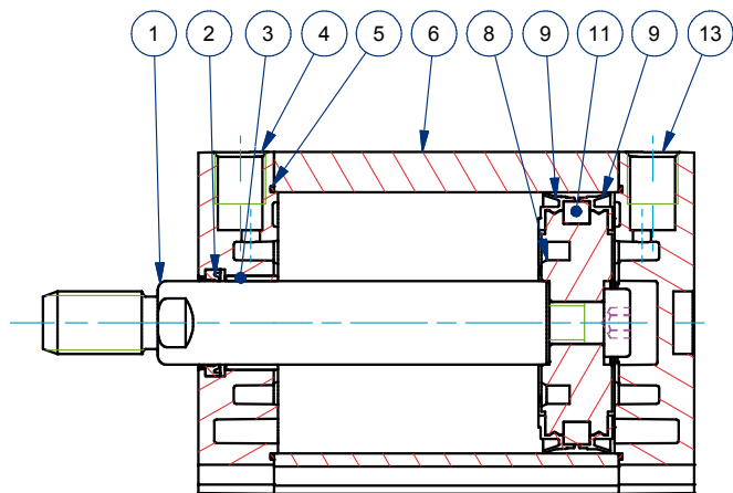
∅32 ÷ ∅125
